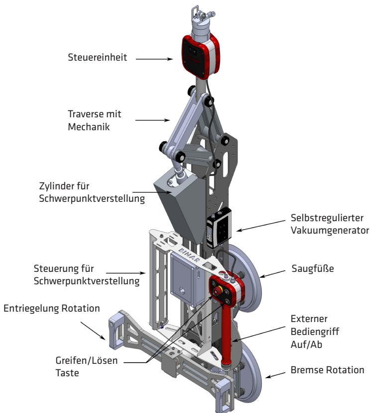
Die Abbildung zeigt ein Lastaufnahmemittel mit manueller Rotation.
